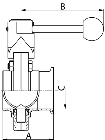
43101 - Csatlakozás : Hegeszthető / Clamp (S-C)
