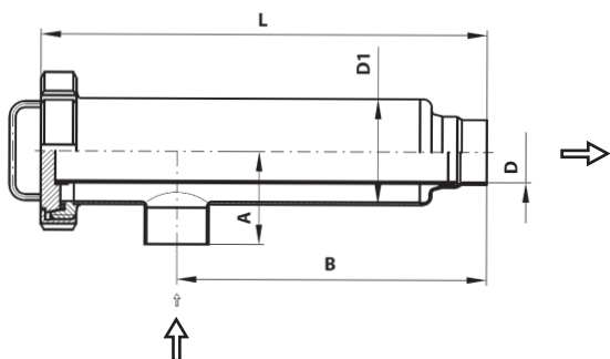
Csőszűrő S-S (hegeszthető-hegeszthető)
