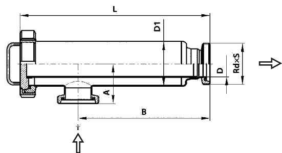
Csőszűrő G-G (menetes-menetes)
